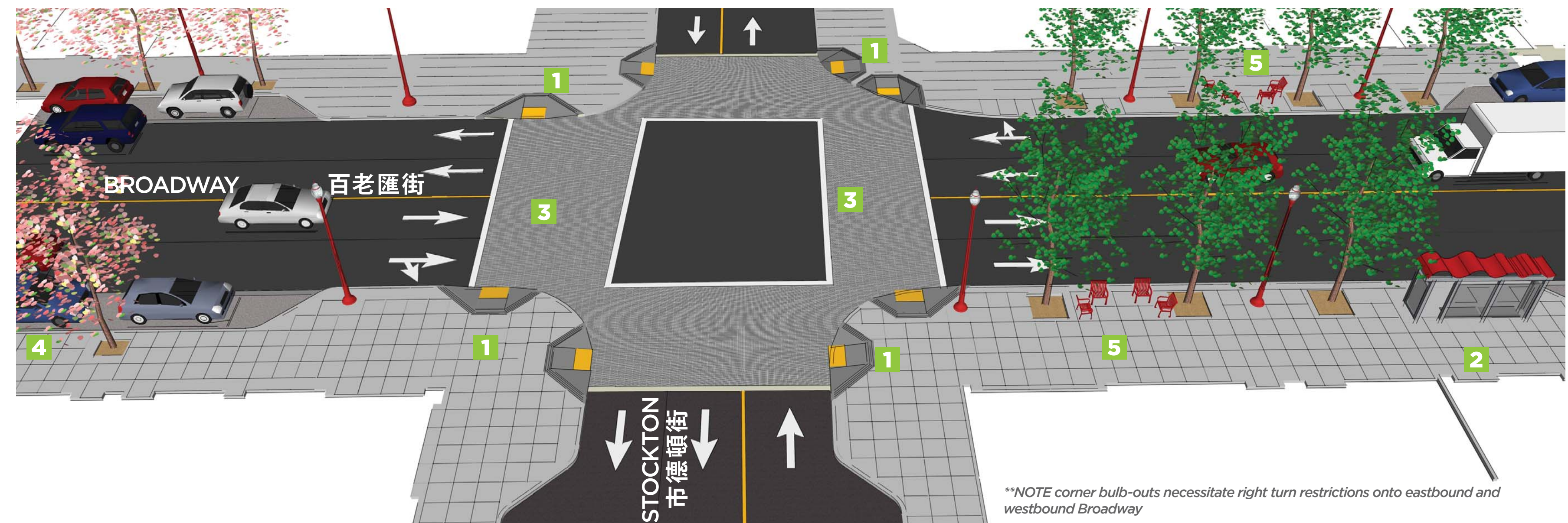
2 BUS STOP IMPROVEMENTS 加設有蓋巴士站
