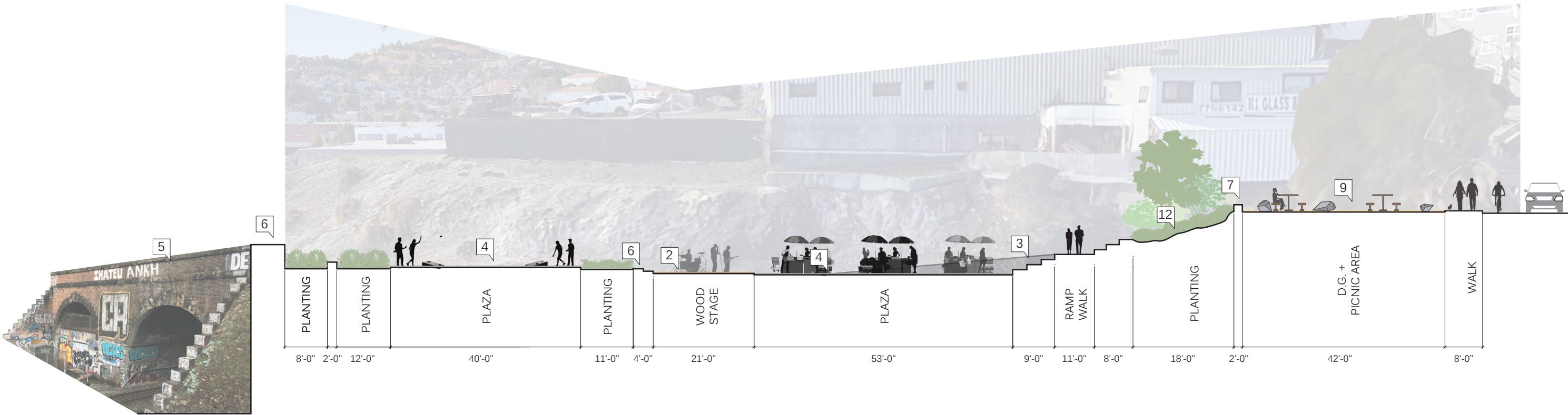
SECTION A-A
