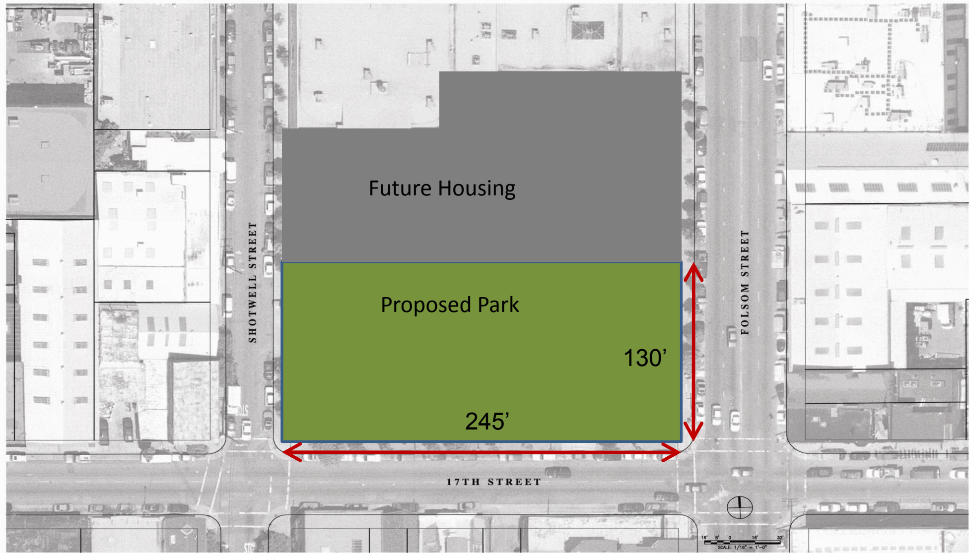
Site Zoning
